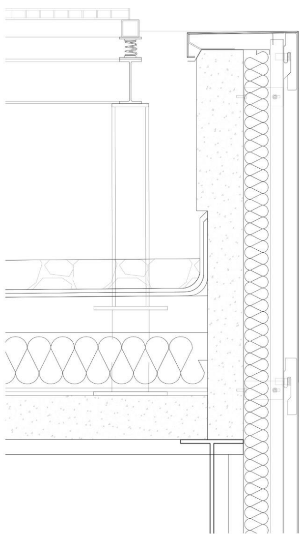
Remate de cubierta
