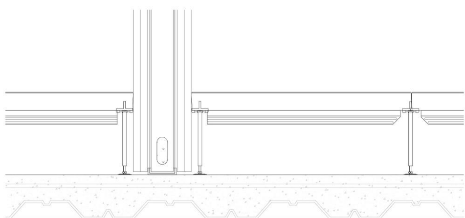
Encuentro suelo técnico con Muros divisorios
