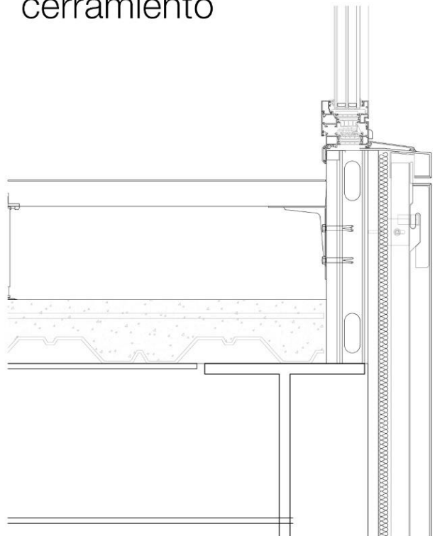
Remate suelo técnico con Cerramiento
