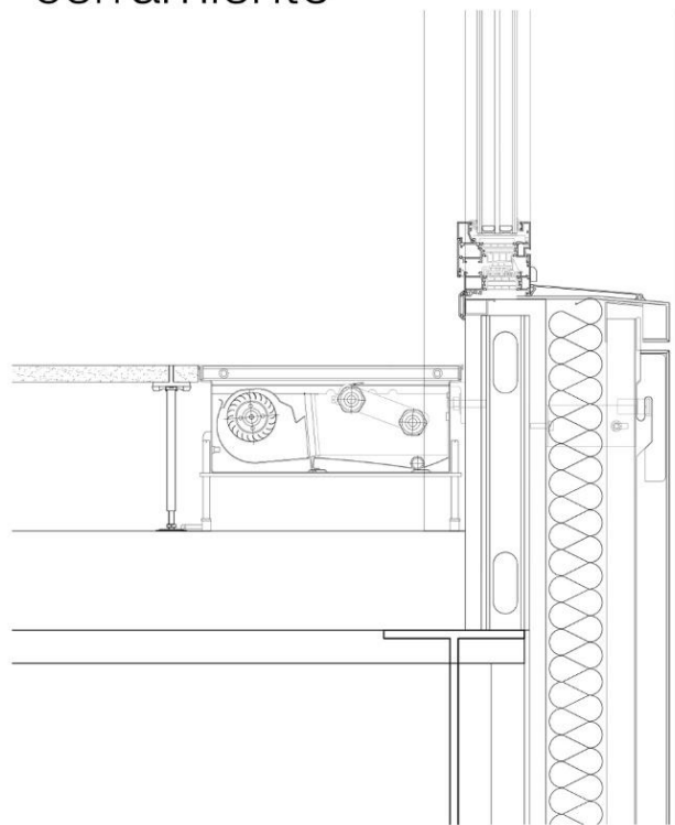
Encuentro de carpintería con cerramiento
