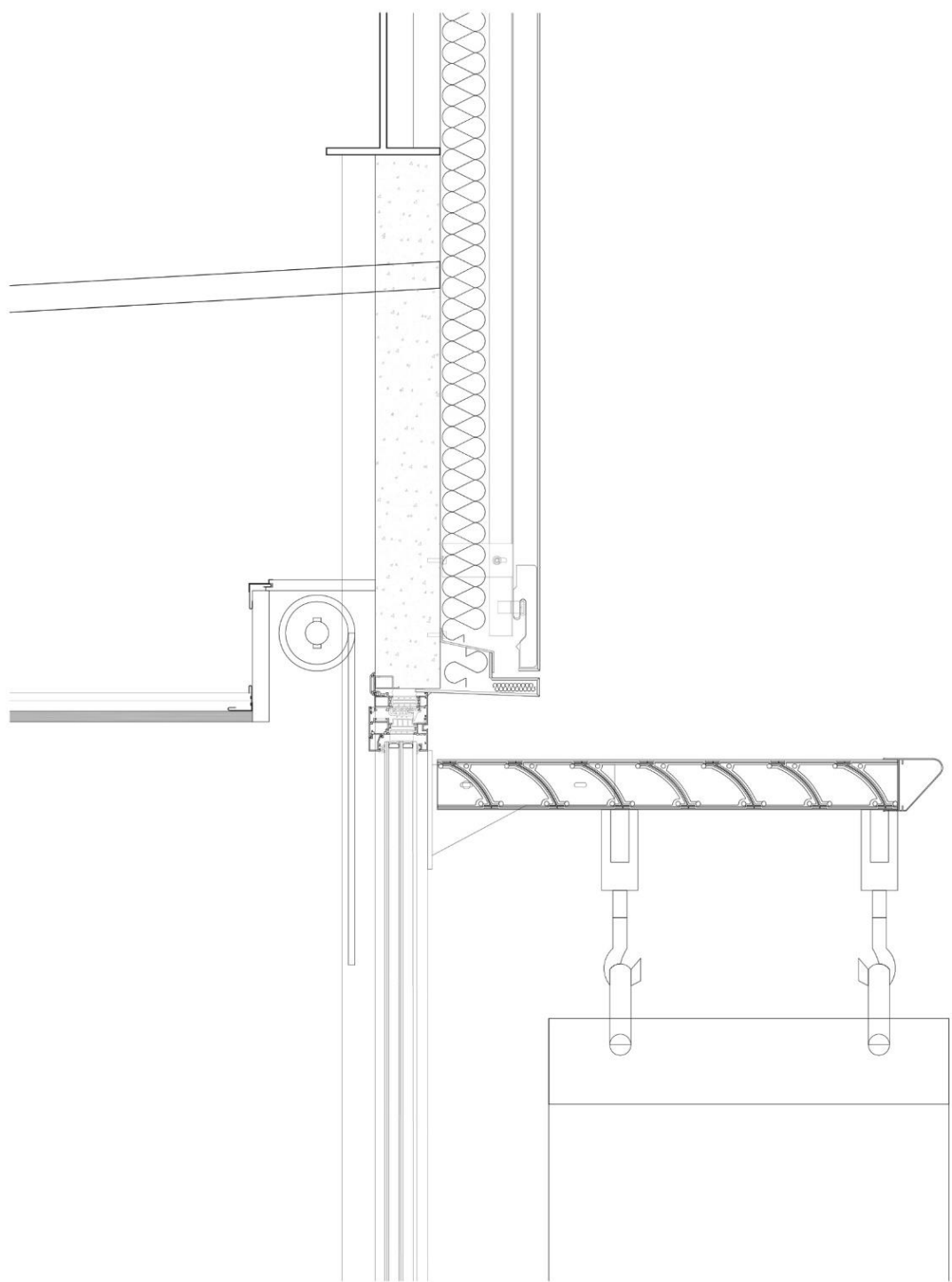
Encuentro de carpintería con cerramiento
