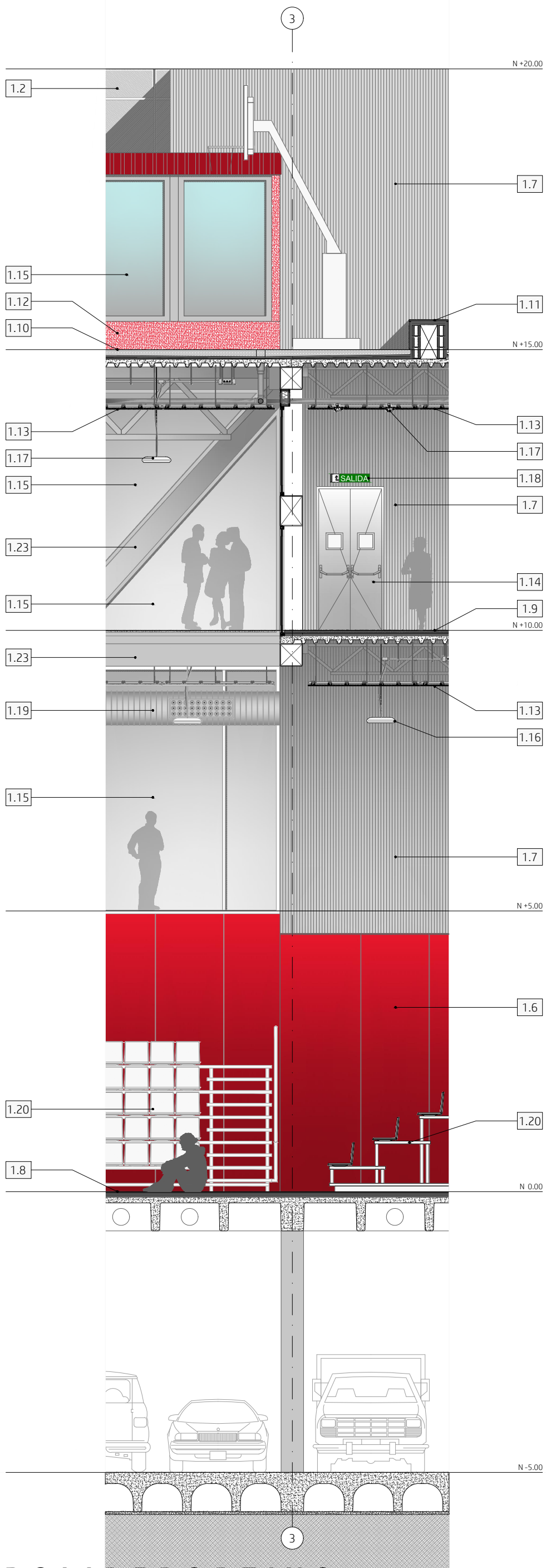
POLIDEPORTIVO GIRARDOTA Detalle Interiores 1 y 2 - Escala 1:75
